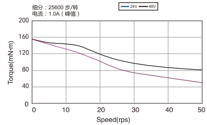
电机力矩曲线
