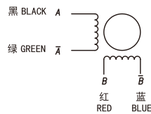
电机接线图
