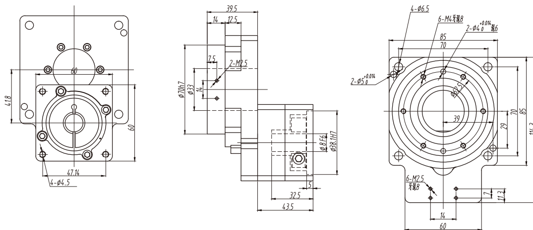
SH85-10-S(尺寸圖)
