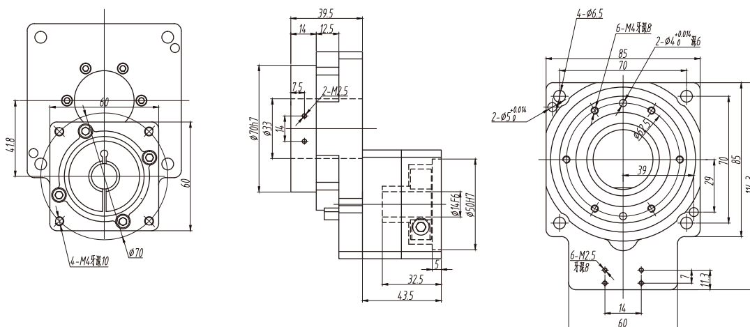
SH85-10-S(尺寸圖)
